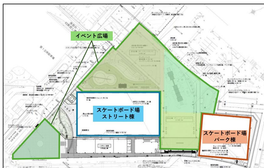
(ボートレース福岡天神ストリートパーク 施設配置図)
